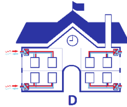
D Mechanische toevoer mechanische afvoer decentraal
